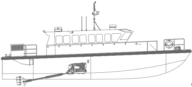
PROFIL
